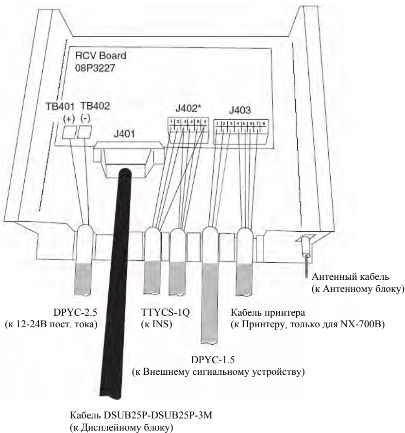
Приемный блок, вид внутри
