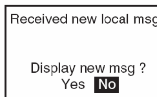
Местное сообщение
