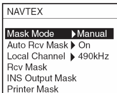
Меню NAVTEX
