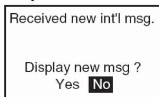
Международное сообщение
